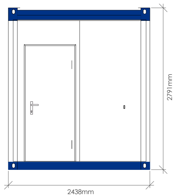
Ansicht A
