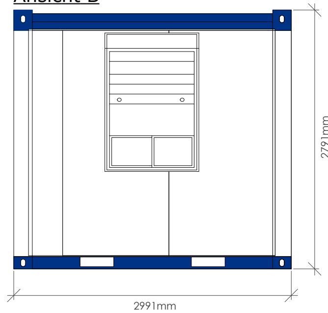
Ansicht D
