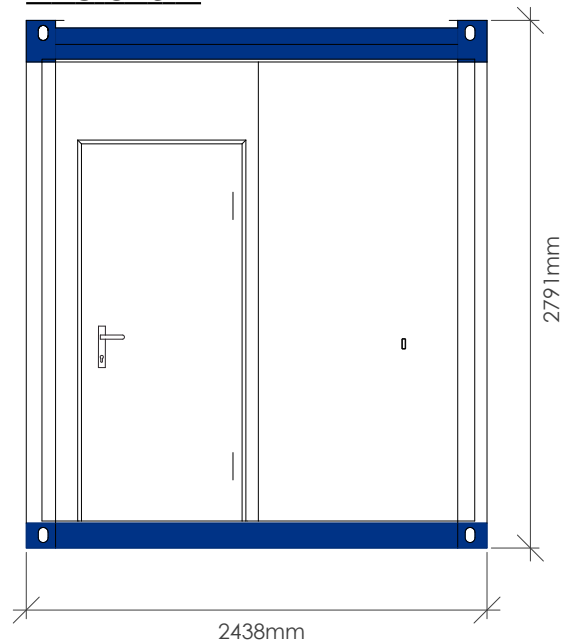
Ansicht C
