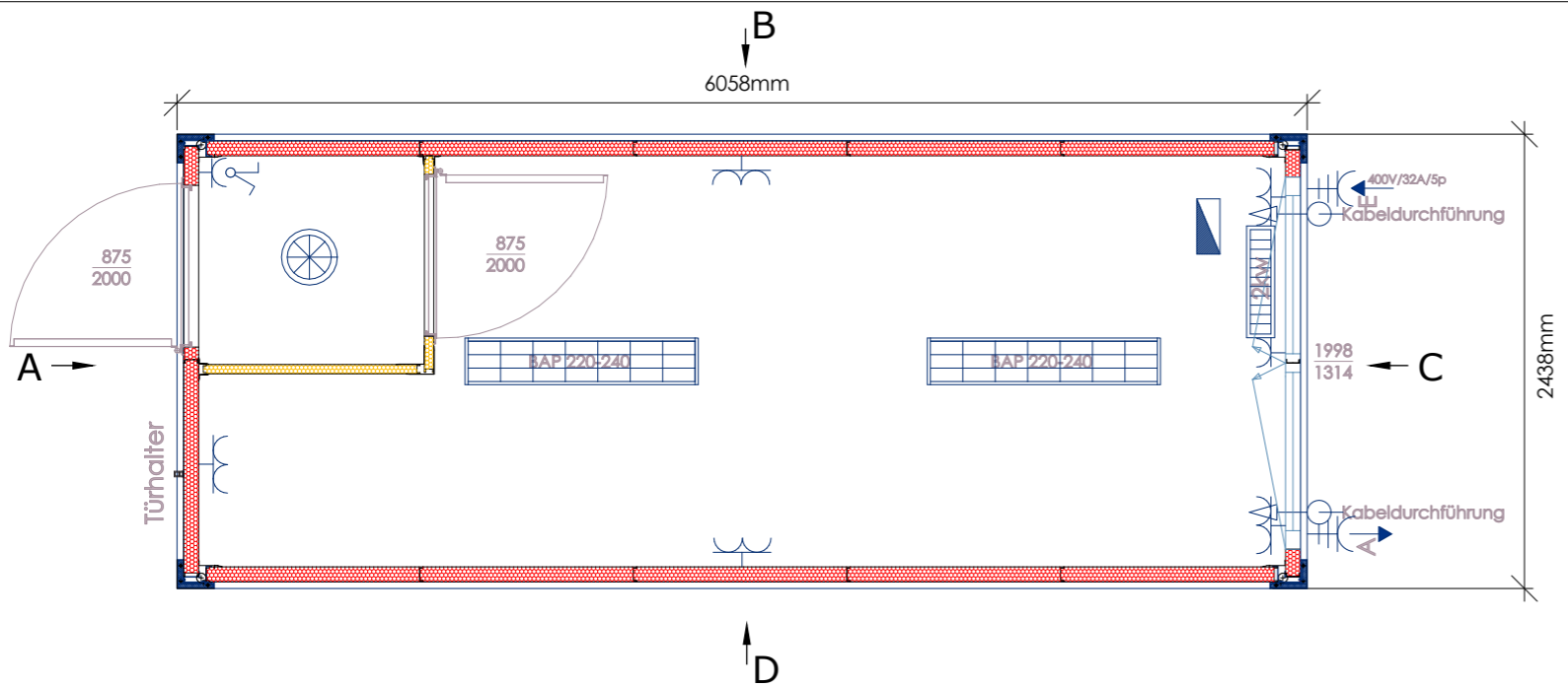
Ansicht A
