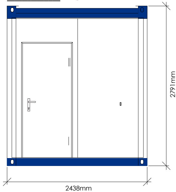
Ansicht A
