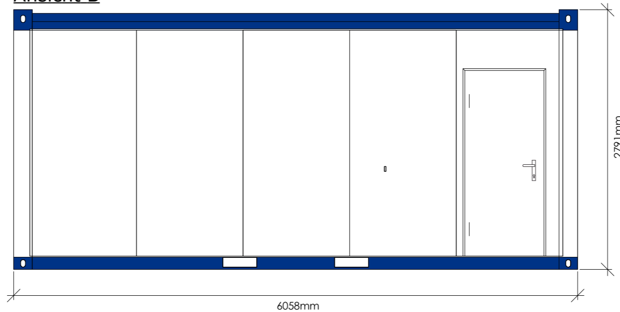
Ansicht B
