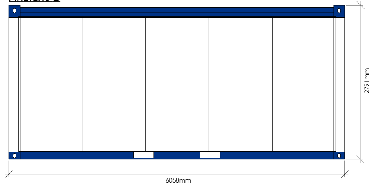
Ansicht B
