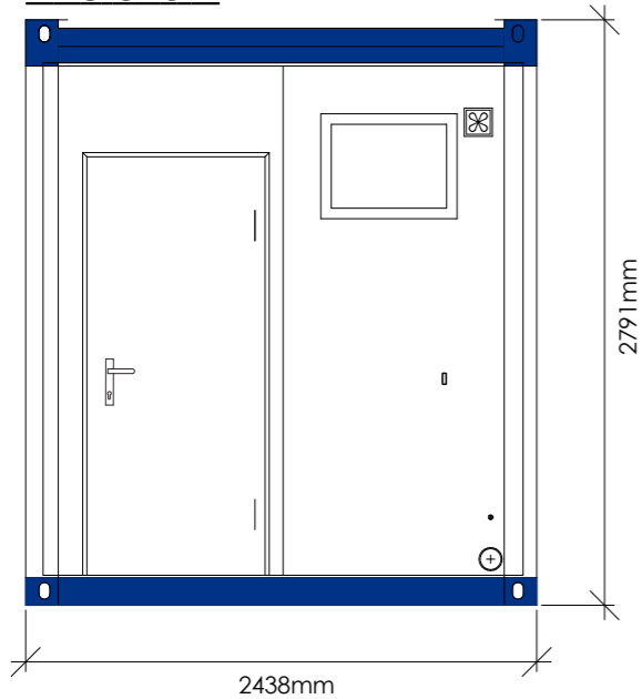
Ansicht A
