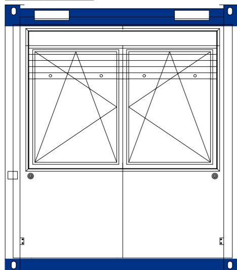
Ansicht C
