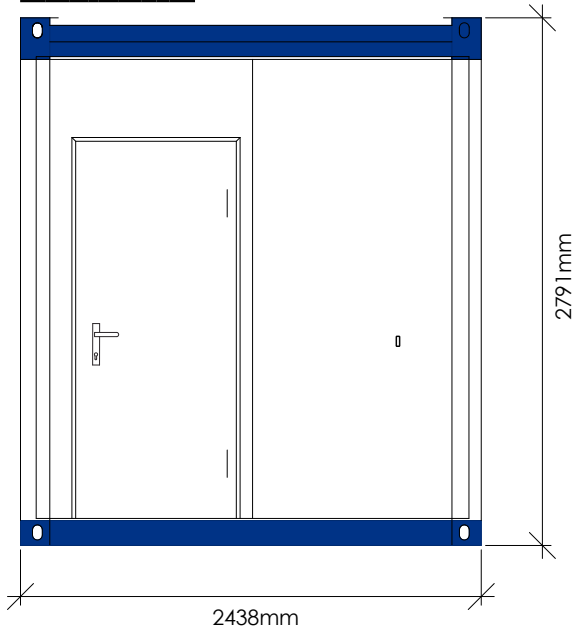
Ansicht A
