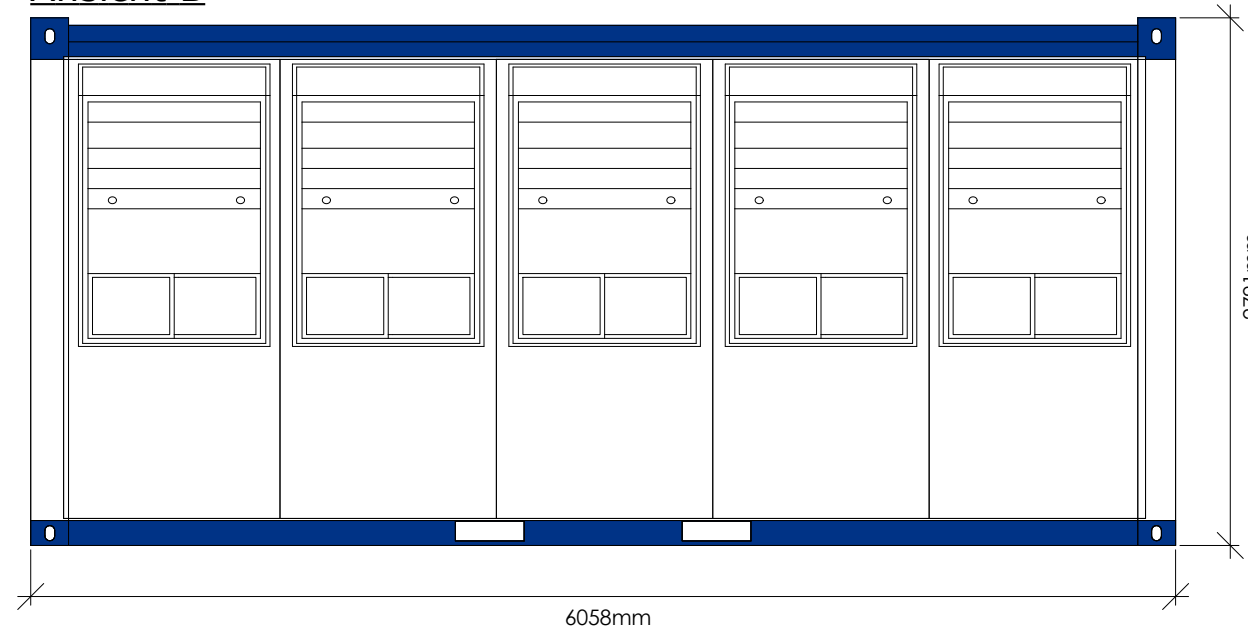
Ansicht B
