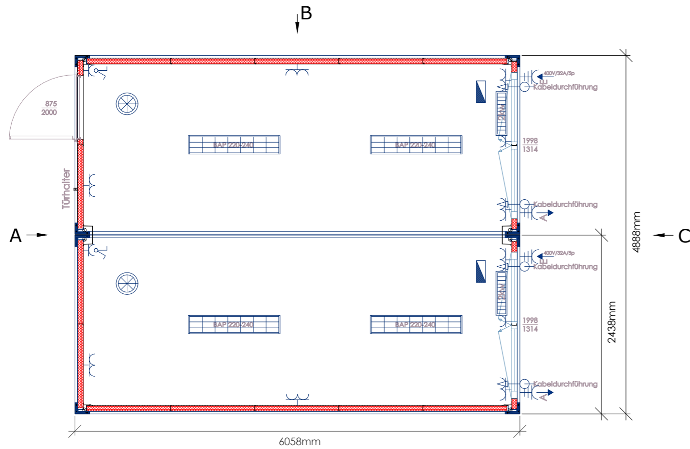
Ansicht A
