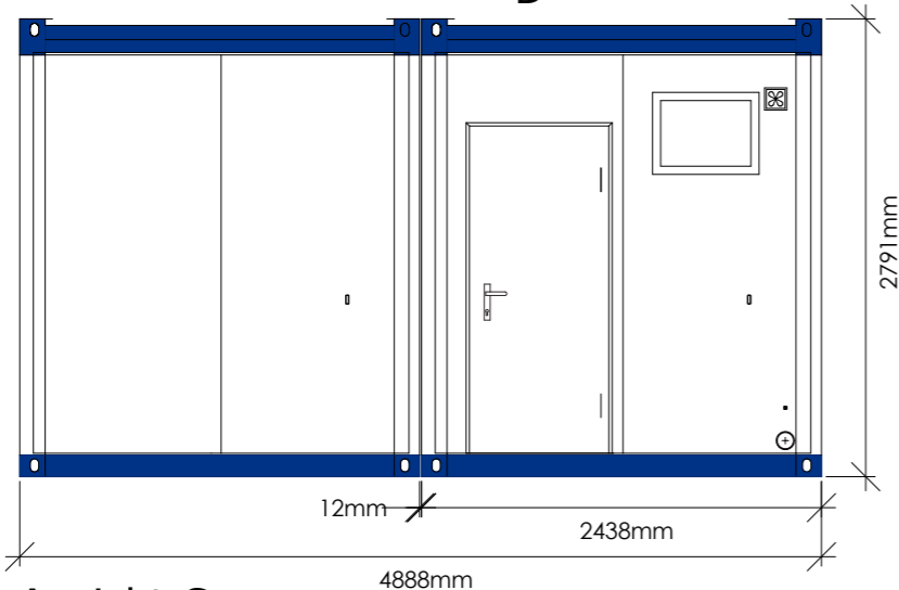
Ansicht C
