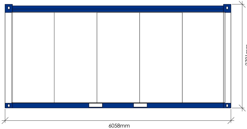
Ansicht D
