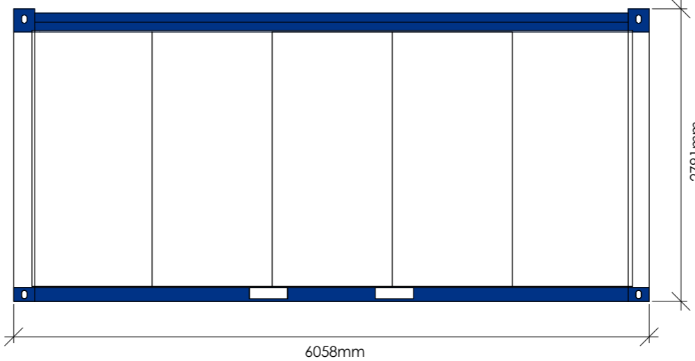
Ansicht D
