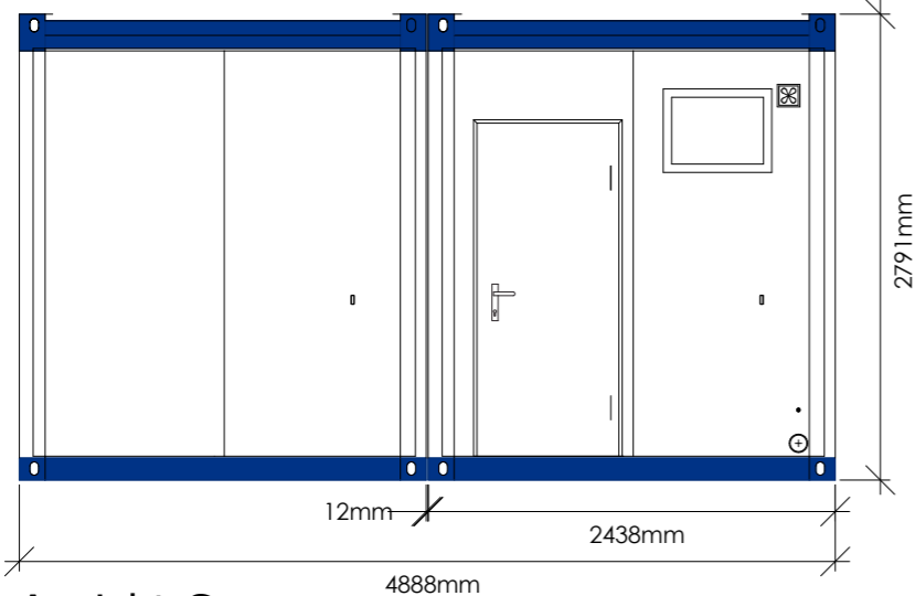
Ansicht C
