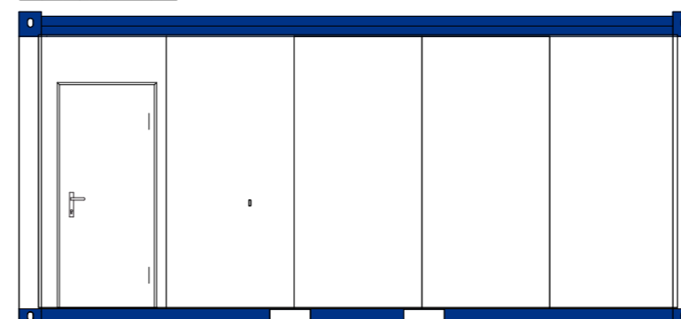
Ansicht D
