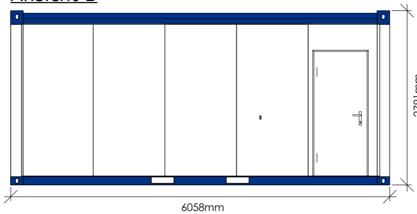
Ansicht D
