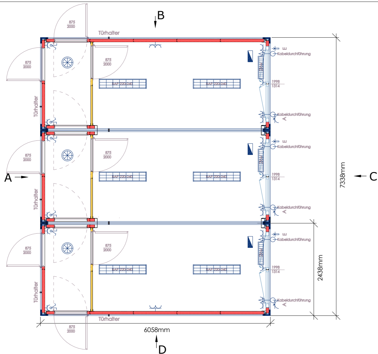
Ansicht A
