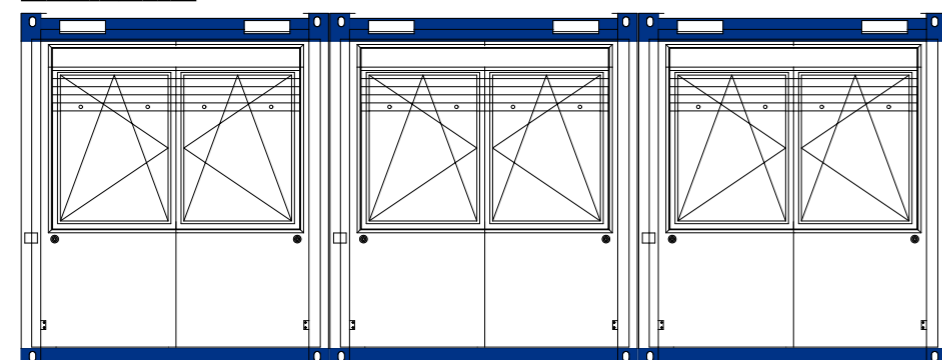
Ansicht C
