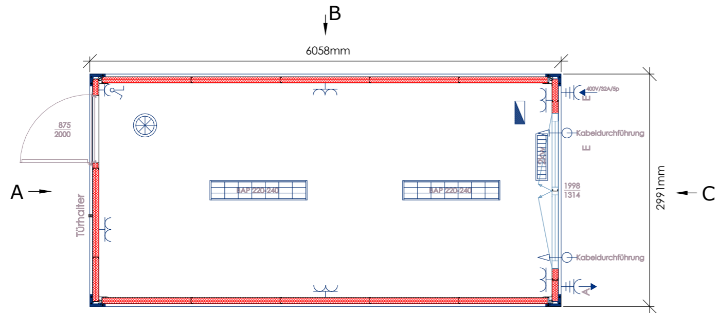
Ansicht A
