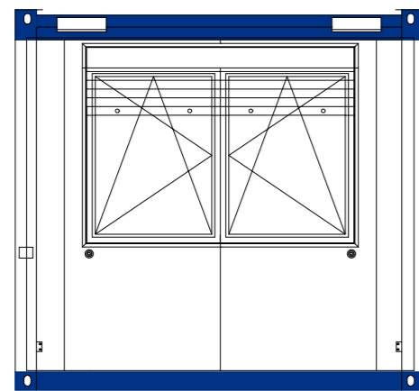
Ansicht C
