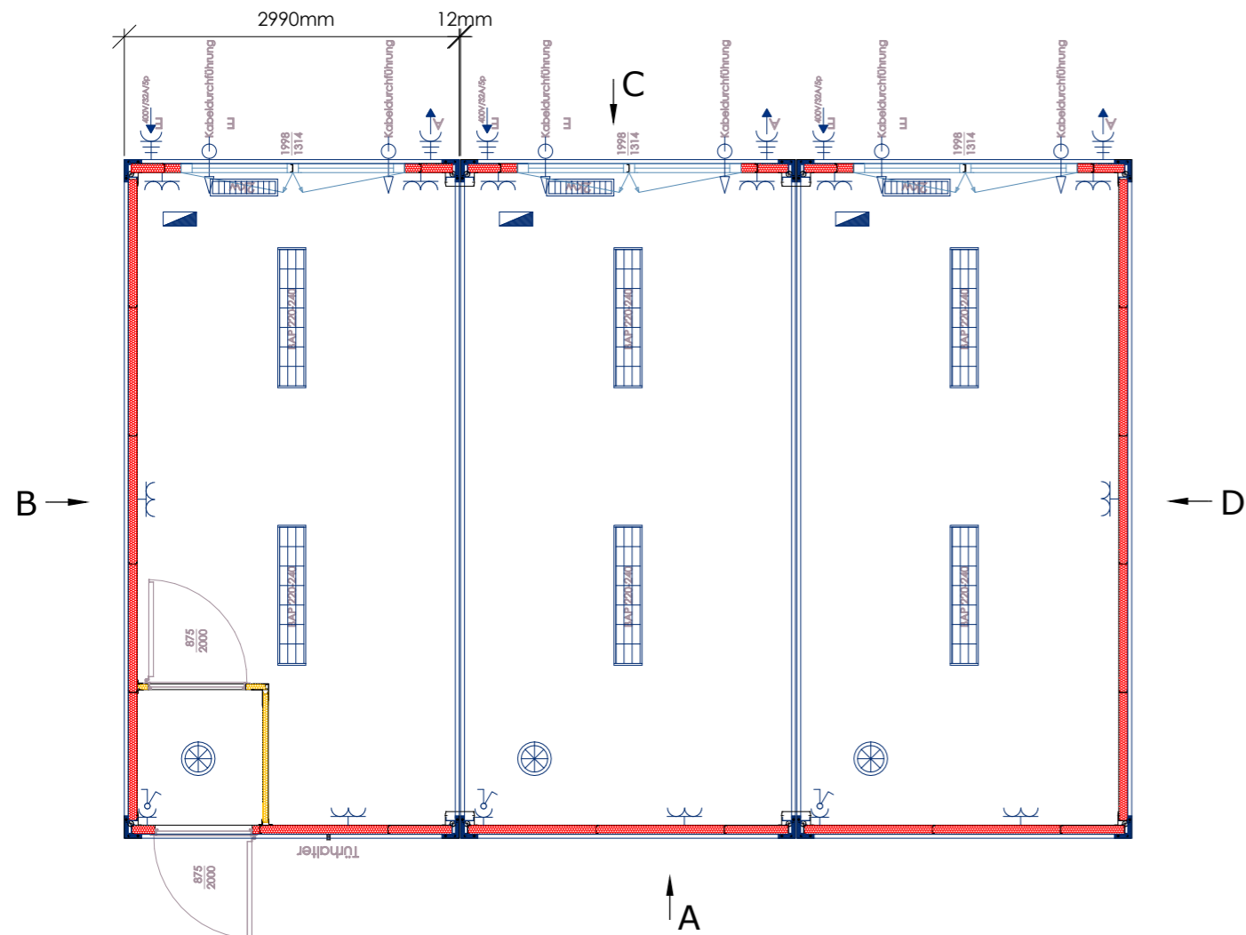
Ansicht A
