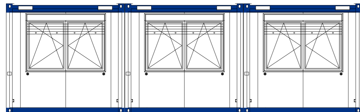
Ansicht C
