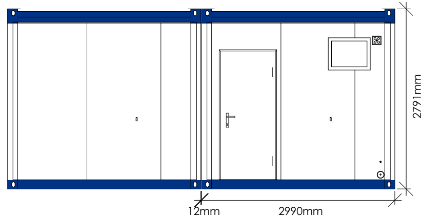
Ansicht C
